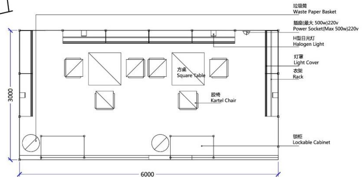
平面图/Floorplan
